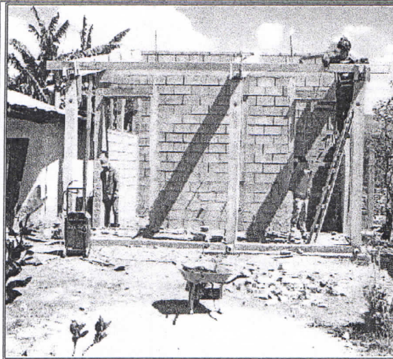
Figure 1 levantamiento de Paredes
