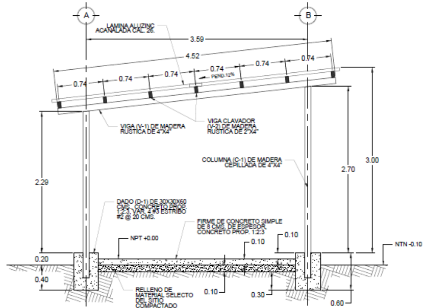
FACHADA LATERAL DERECHA ESCALA: 1/40
