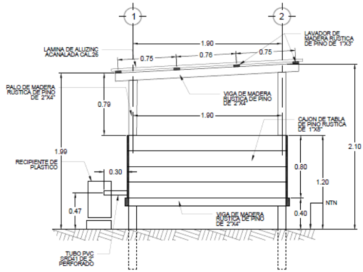
FACHADA LATERAL DERECHA ESCALA: 1/30
