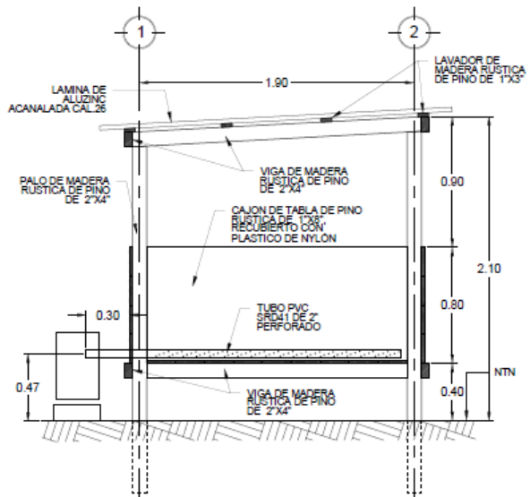
SECCIÓN DE CORTE A-A ESCALA: 1/30
