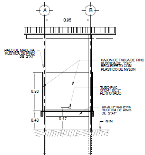
SECCIÓN DE CORTE B-B ESCALA: 1/30
