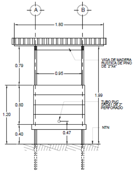
FACHADA FRONTAL ESCALA: 1/30
