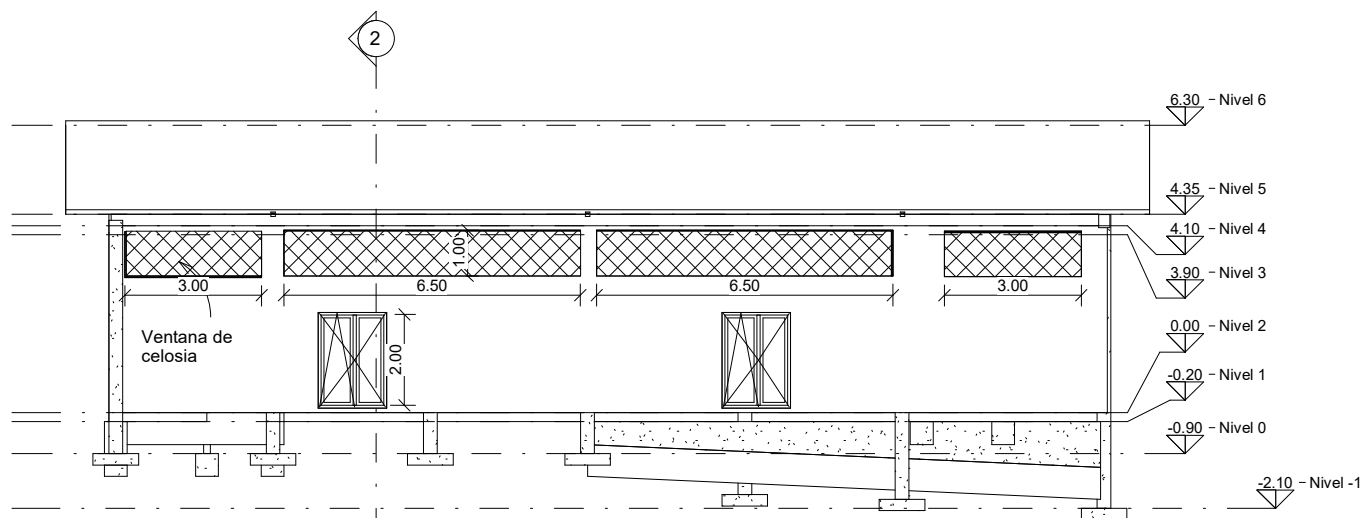
1 Oeste A106 1:100
