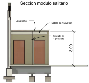
3 Sección 5 A104 1: 100
