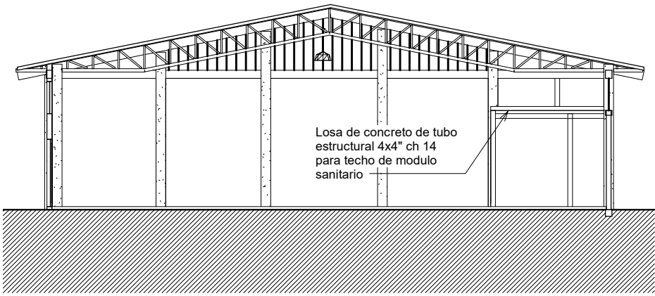
2 Sección 9 A104 1: 100
