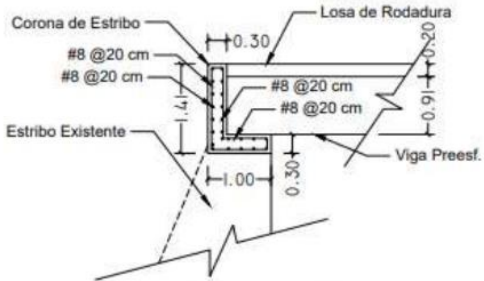
DETALLE DE CORONA DE ESTRIBO
