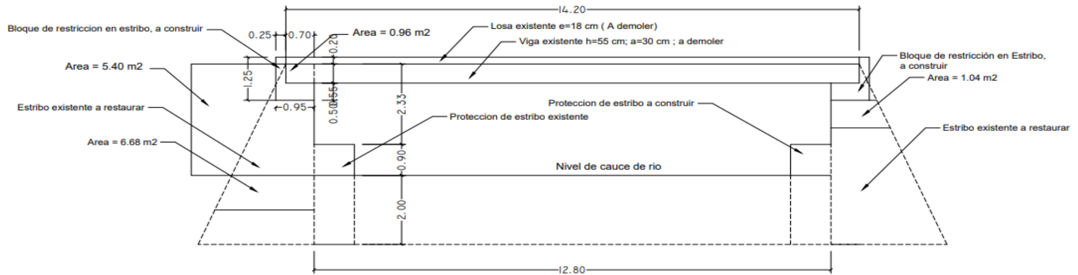
VISTA LATERAL PUENTE
