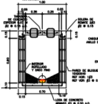
SECCION A - A CAJA POZO SIN ESCALA
