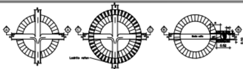
POZO DE INSPECCION h < 3.50 SIN ESCALA
