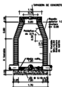
CORTE A - A POZO DE INSPECCION h < 3.50 SIN ESCALA
