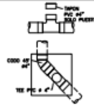
SISTEMA SELLADO CAJA DOMICILIARIA SIN ESCALA
