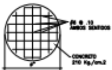
ARMADO DE TAPADERA SIN ESCALA
