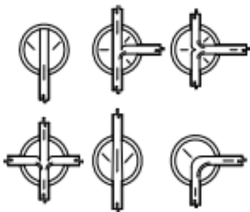
MEDIAS CAÑAS CON ACABADO FINO DE CEMENTO, CASOS TÍPICOS DE POZO SIN ESCALA
