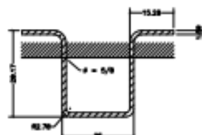
PEDAÑO DE POZO SIN ESCALA DIMENSIONES EN CM
