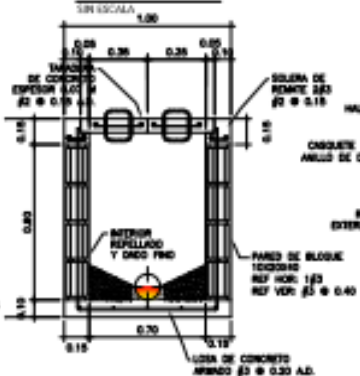
SECCION A - A CAJA POZO SIN ESCALA
