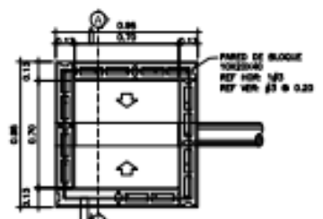
PLANTA CAJA POZO SIN ESCALA
