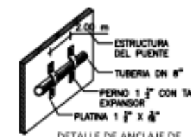
DETALLE DE ANCLAJE DE TUBERIA EN PUENTE SIN ESCALA
