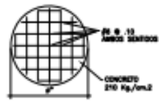
ARMADO DE TAPADERA SIN ESCALA
