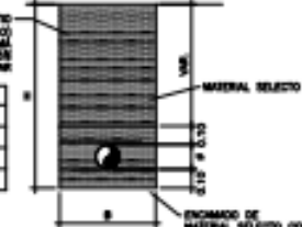
DETALLE DE ZANIAS SISTEMA DE AGUAS NEGRAS SIN ESCALA
